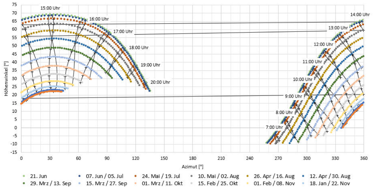
Reflexionsdiagramm der Modulfläche (UTC+1) bei Westausrichtung
