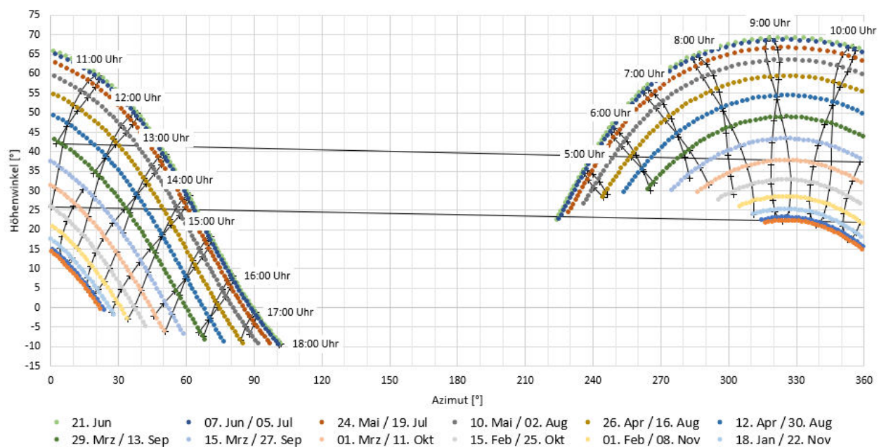
Reflexionsdiagramm der Modulfläche (UTC+1) bei Ostausrichtung
