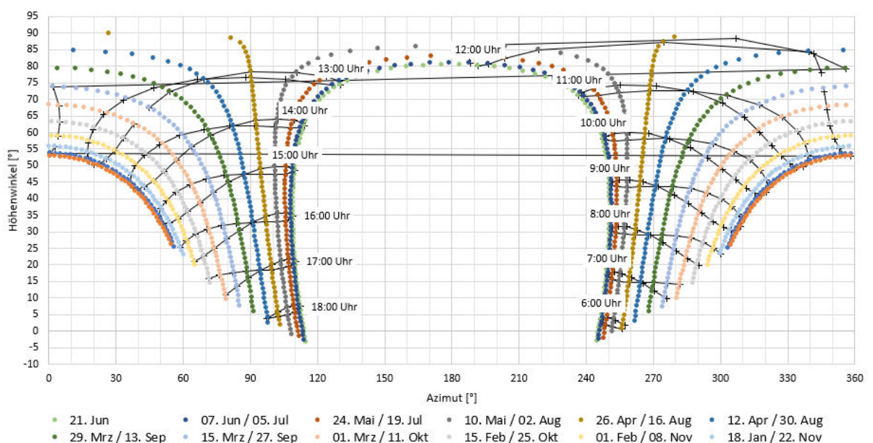
Reflexionsdiagramm der Modulfläche (UTC+1) bei Südausrichtung
